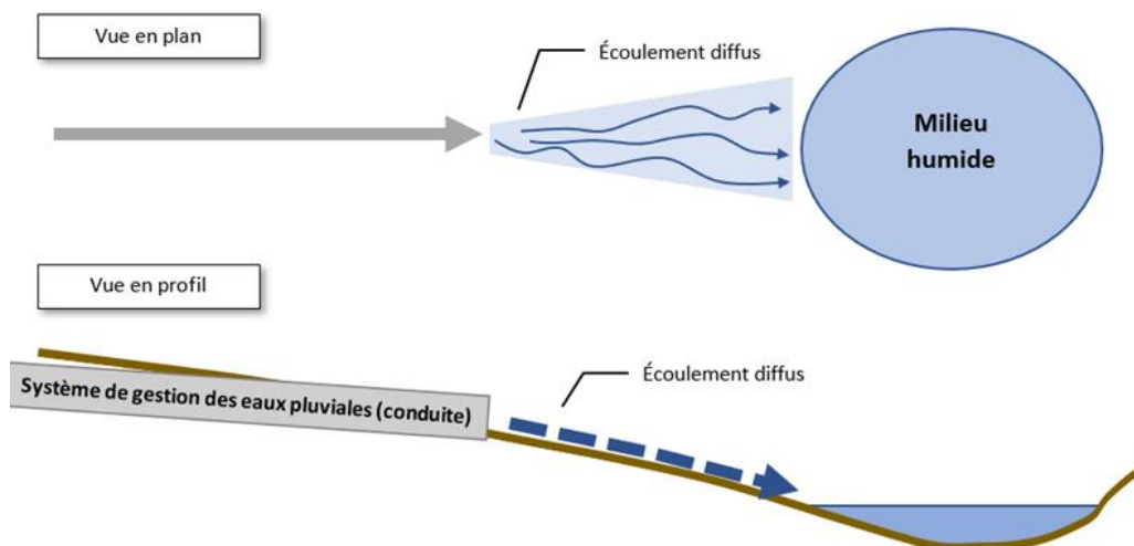
Figure 222.2 Écoulement en surface atteignant un milieu humide (cas d'un écoulement diffus)
