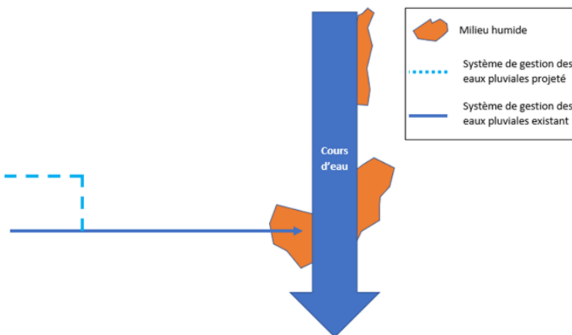
Figure 222.4 Situation où la condition 4 est satisfaite lorsqu'il s'agit d'un milieu humide localisé dans la rive ou le littoral d'un cours d'eau.
