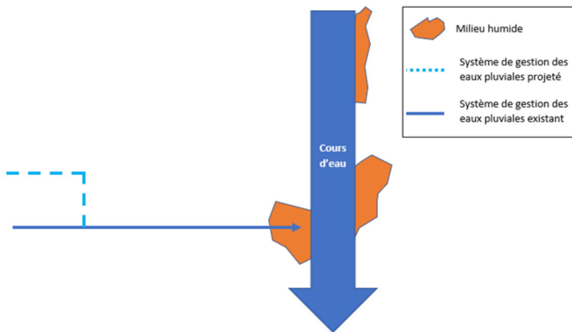
Figure 224.6 Situation où la condition 5° est satisfaite lorsqu'il s'agit d'un milieu humide localisé dans la rive ou le littoral d'un cours d'eau.
